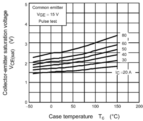
Fig. 8.5 VCE(sat) - Tc
