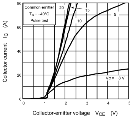
Fig. 8.1 IC - VCE
