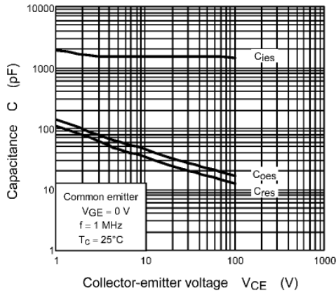
Fig. 8.8 C - V_{CE}
