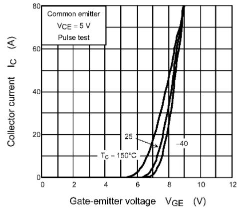
Fig. 8.6 IC - VGE
