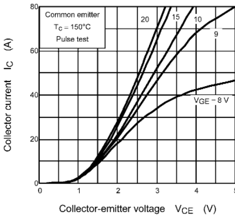
Fig. 8.3 IC - VCE
