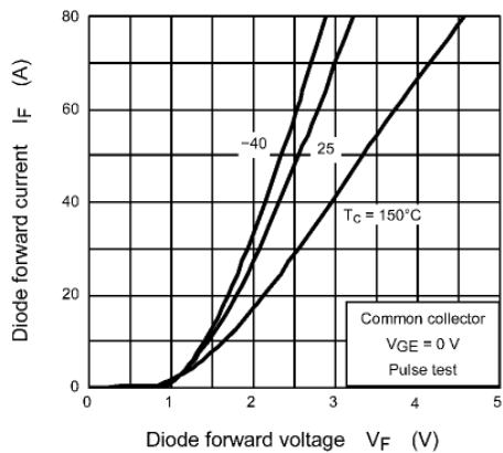
Fig. 8.14 I_F - V_F
